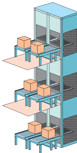
垂直仕分搬送機
